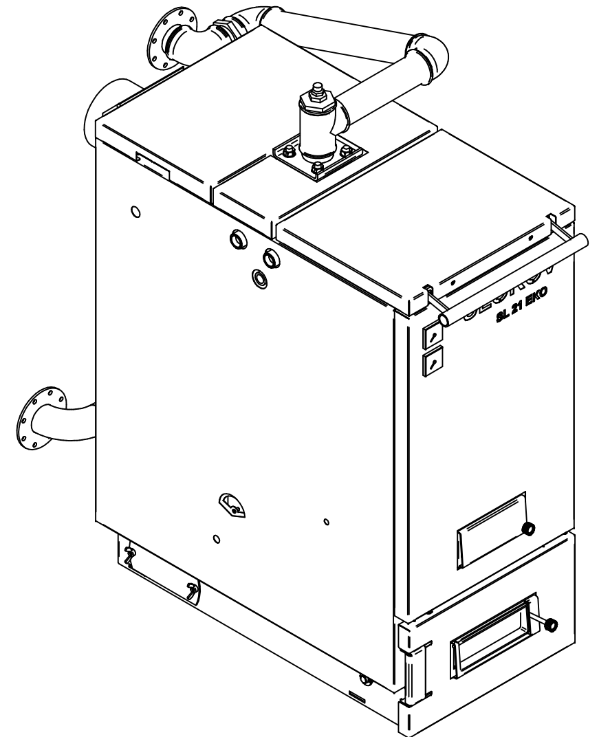
KOTEL SL21EKO S PŘESTAVBOVOU SADOU č.2
