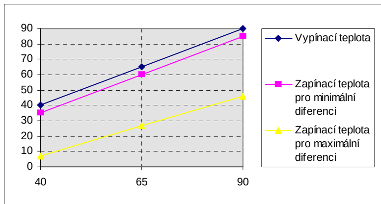
obr. 1 Rozsah nastavení difference mezi vypínací a zapínací teplotou
