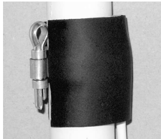
Izolace čidla termo- izolační páskou
